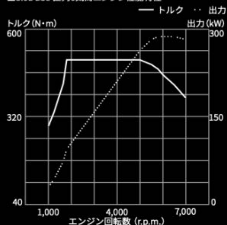
■3.0L B58 直列6気筒エンジン性能特性
