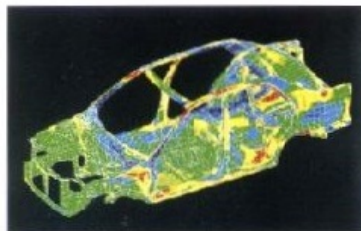
ตัวถังแบบโมโนค็อก (Monocoque)
