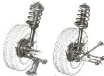
ระบบกันสะเทือนอิสระทั้ง 4 ล้อ ให้สมรรถนะการทรงตัวและความนุ่มนวลขณะขับเคลื่อน
